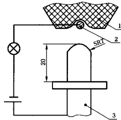
图 1 手柄结构测试
