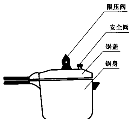
图 A.1 旋合式结构示意图
